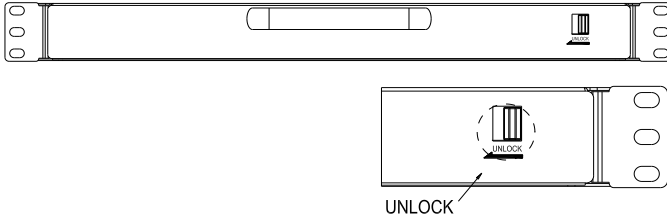
图 3-3 解锁方式
