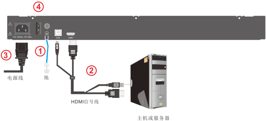
图 3-2 连线方式
